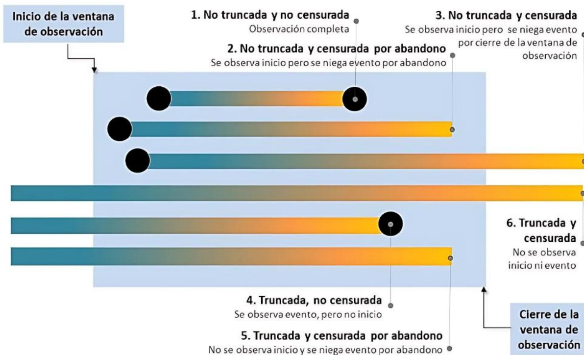
Figura 1 Tipos de observación por modelo de truncamiento o de censura
