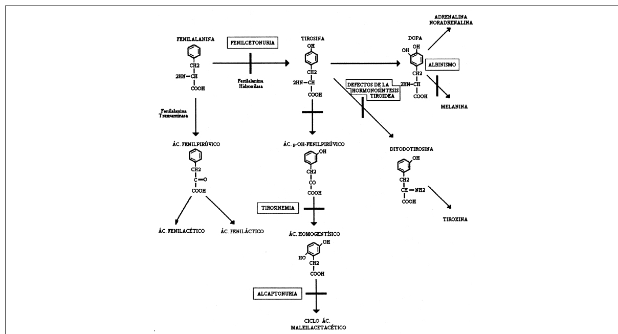
Figura 1. Metabolismo de la fenilalanina y sus derivados
