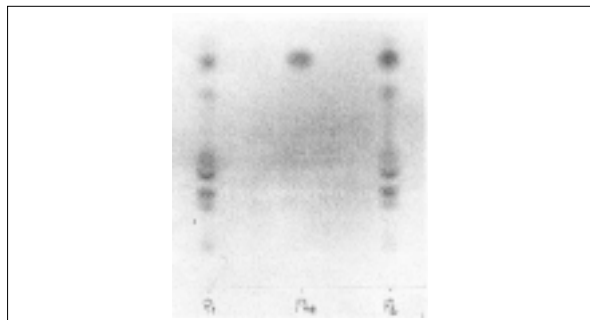
Figura 3. Cromatografía para aminoácidos en sangre
